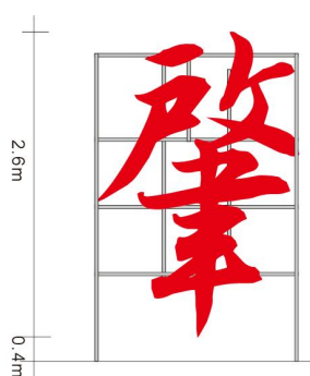
正视图
